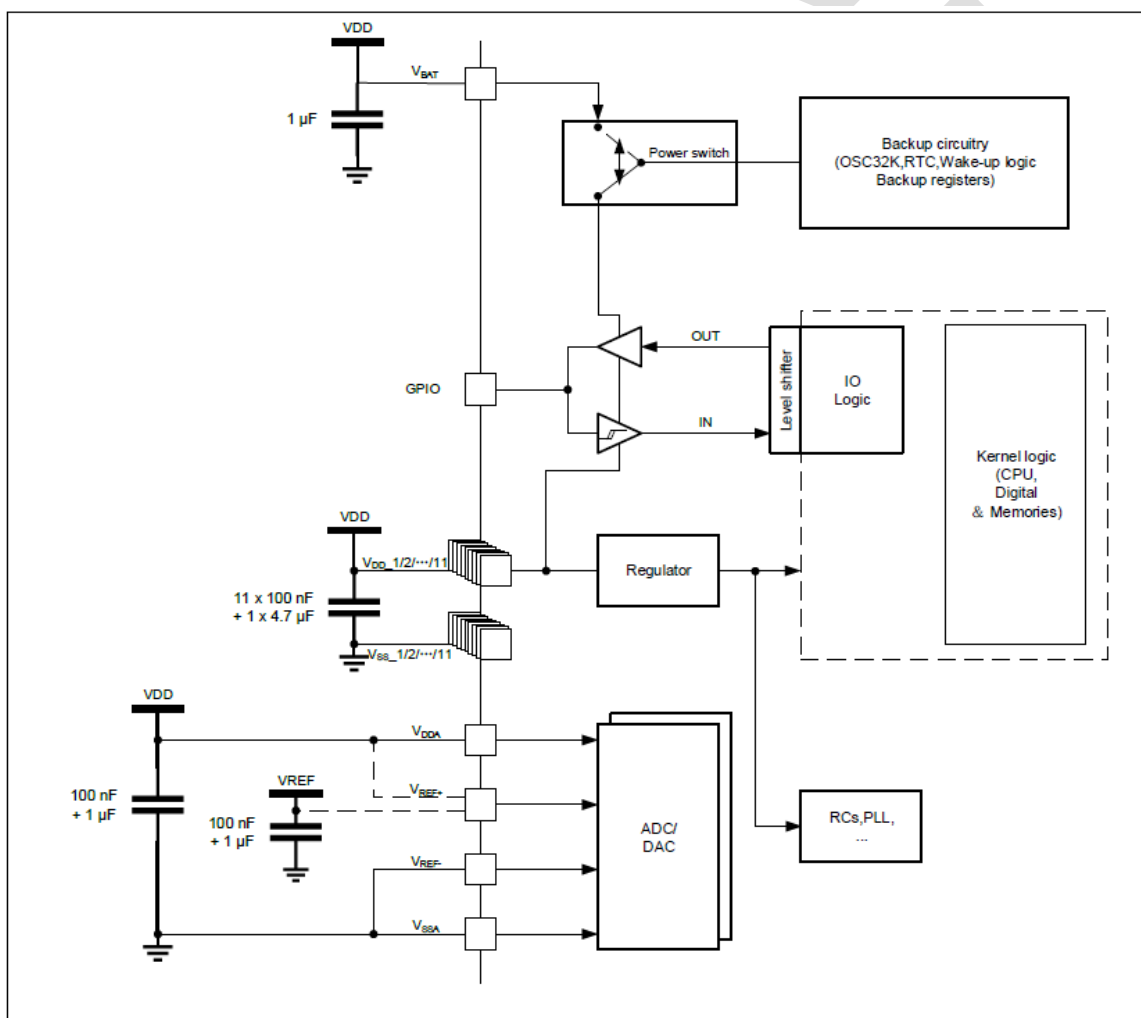
图 5 供电方案
