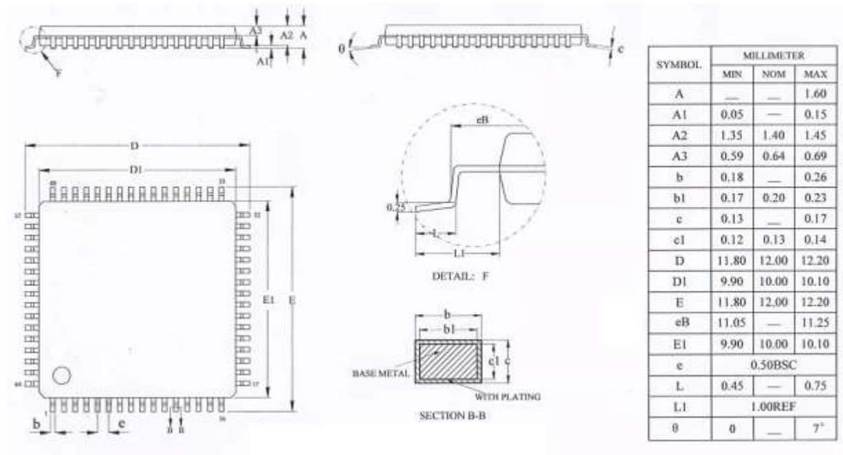
图 15 LQFP64 10mm×10mm封装尺寸
