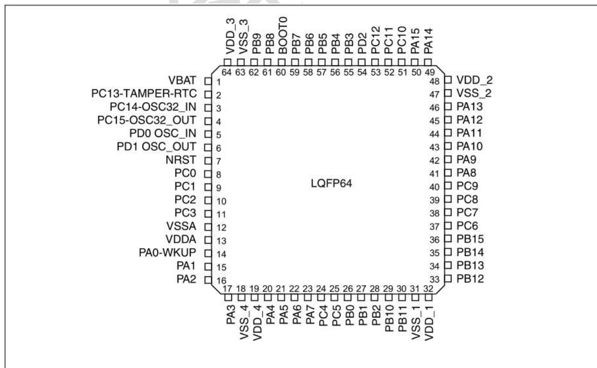
图 2 LQFP64封装
