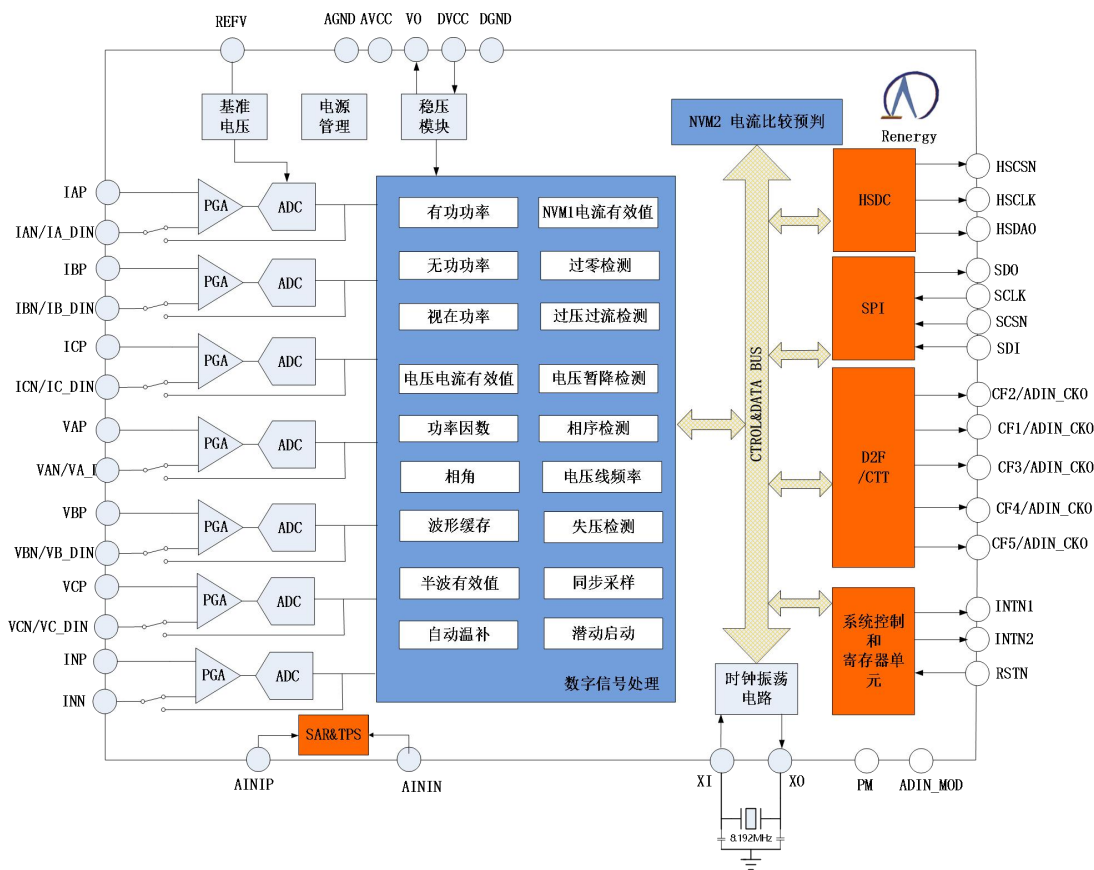
图 1-1 系统框图
