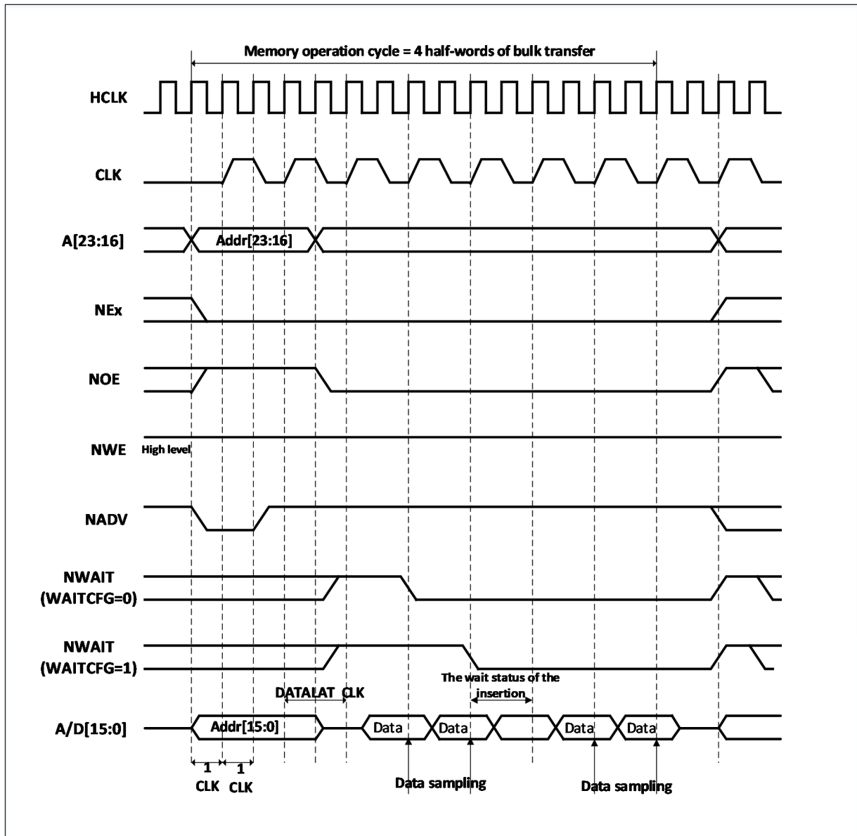
图 26-13 同步总线复用读操作（复用）
