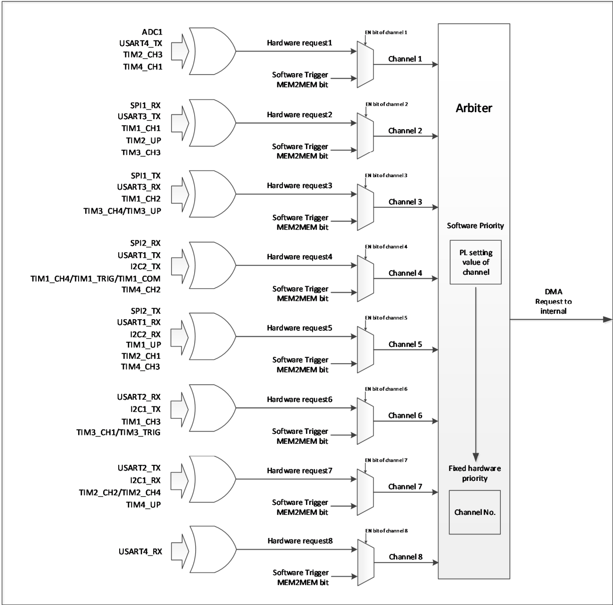
图 11-3 DMA 请求映像
