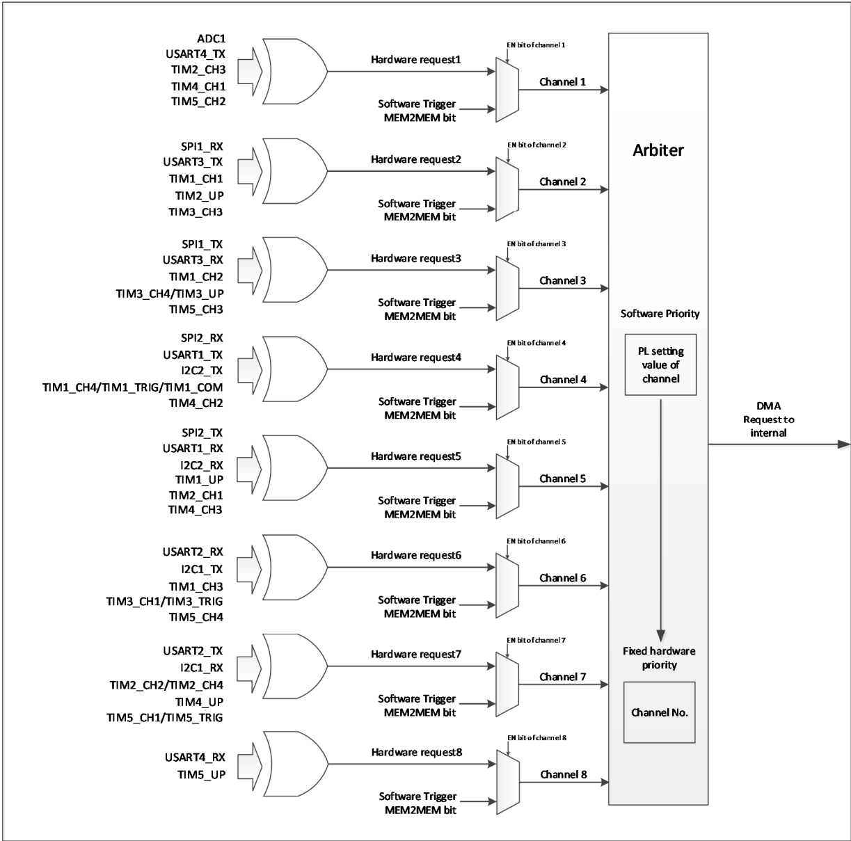
图 11-4 DMA 请求映像
