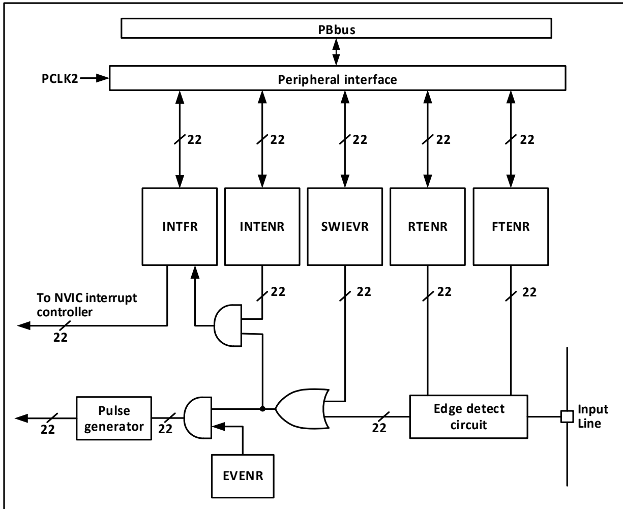
图 9-1 外部中断（EXTI）接口框图
