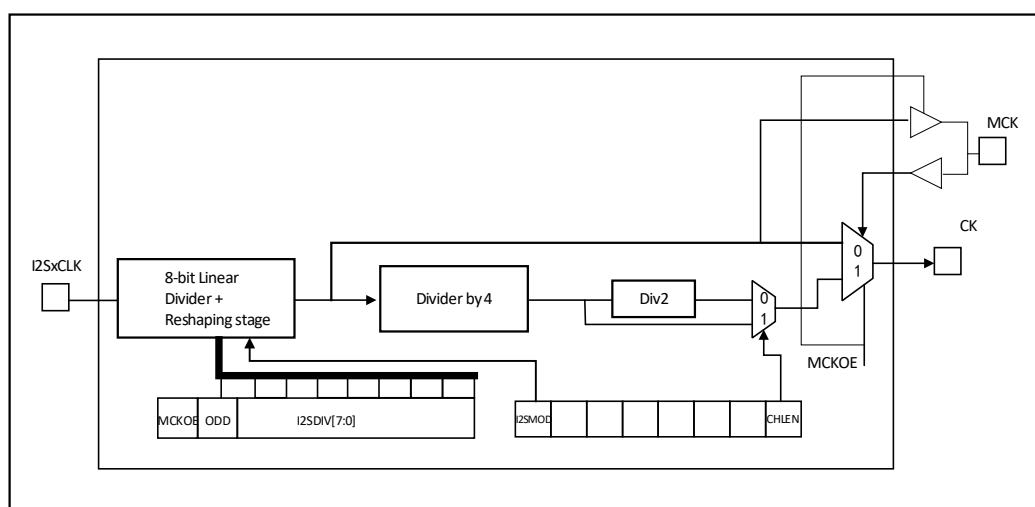
图 20-16 12S 时钟发生器结构
