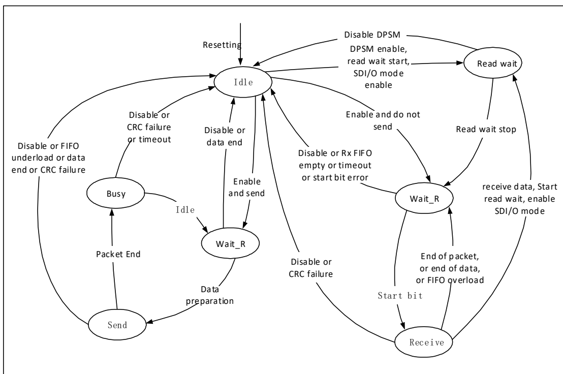
图 28-3 数据状态机
