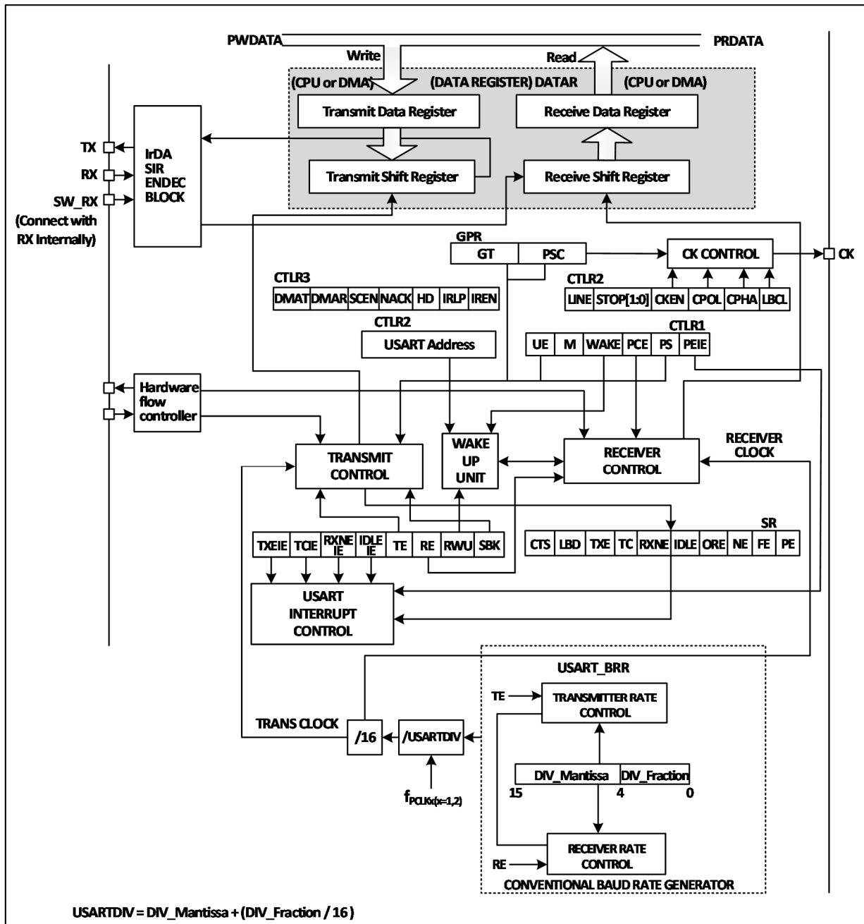
图 18-1 通用同步/异步收发器的结构框图
